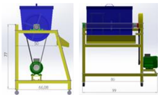
Gambar 2. Rancangan mesin pengaduk adonan ampiang
